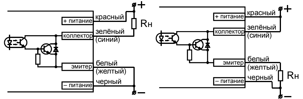
Рис.2. Схемы подключения фотодатчика МикРА Ф2Б.
