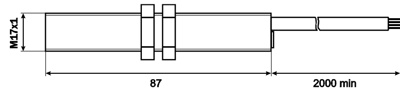
Рис.1. Габаритные размеры фотодатчика МикРА Ф2Б.
