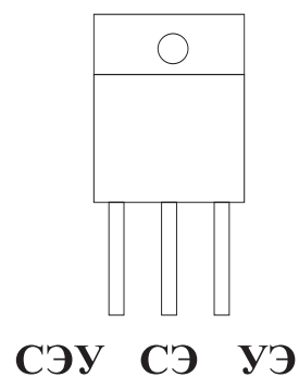
Расположение выводов симисторов BT139-600, BTV16-6, BTA41-600
