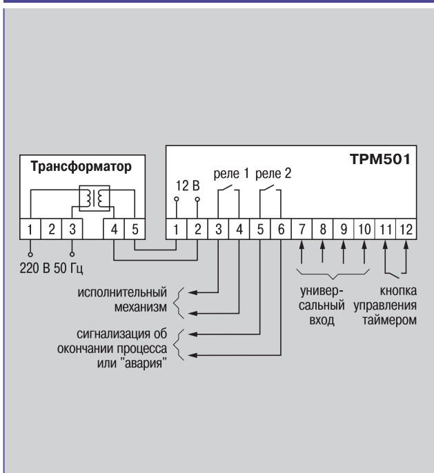
▲ Общая схема подключения TRM501
