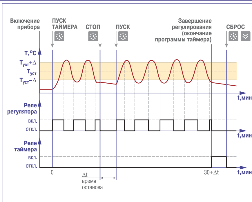
▶ Пример работы TRM501 в режиме регулирования по таймеру (режим 1)
