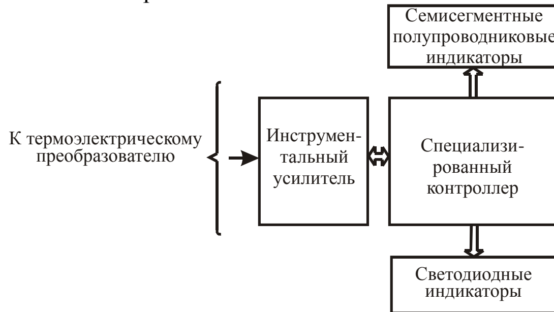
Рисунок 3.1 – Функциональная схема прибора
