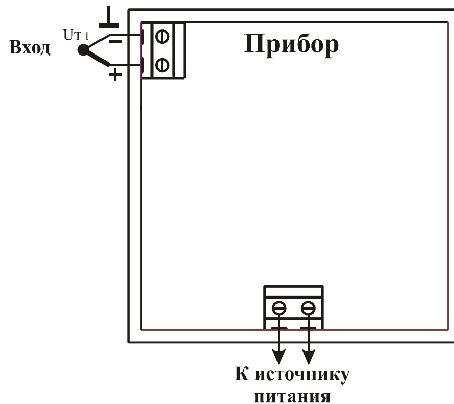
Рисунок 8.1 – Схемы подключения ПТ и источника питания
