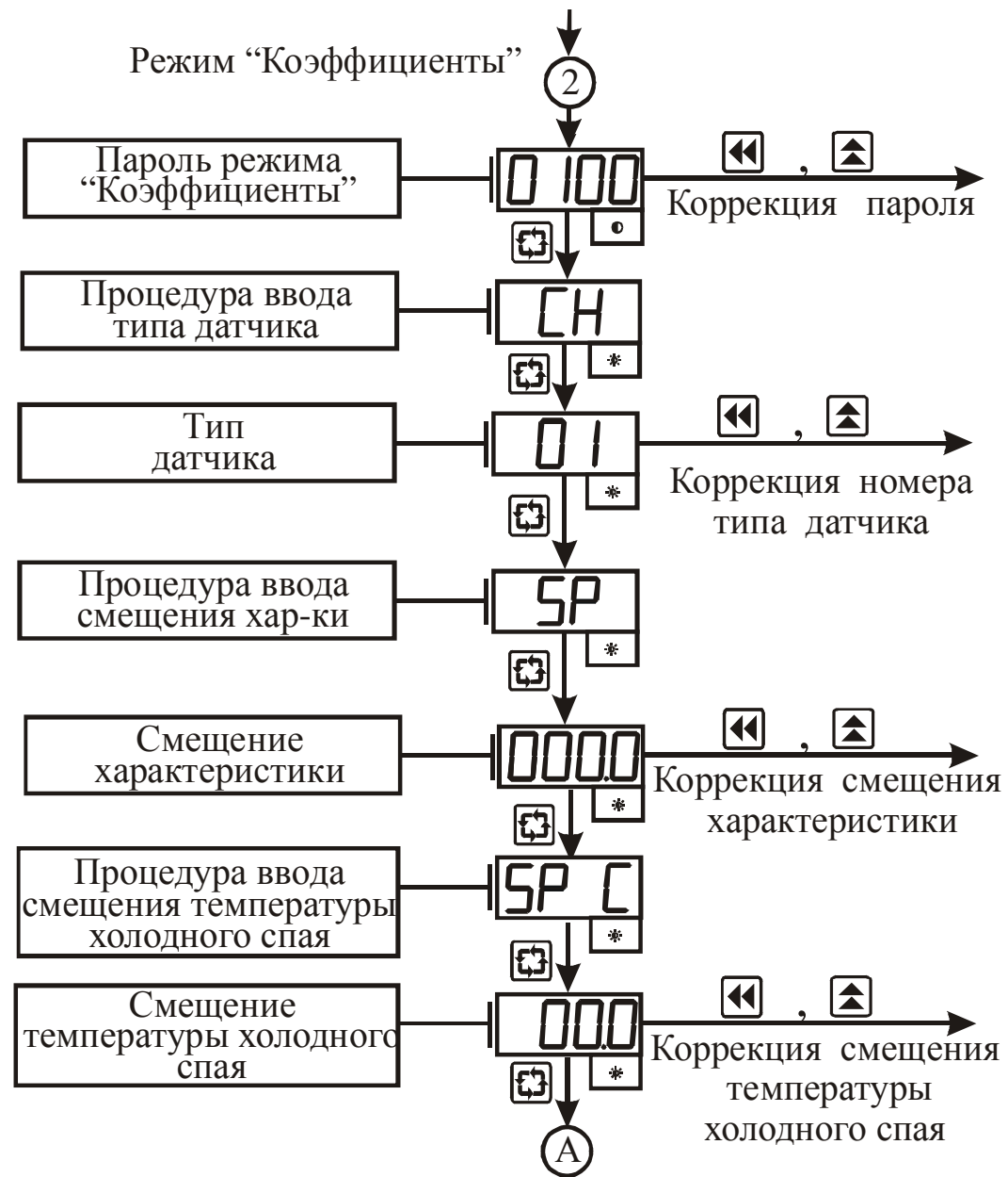
Рисунок 3.4 – Схема алгоритма работы в режиме “Коэффициенты”
