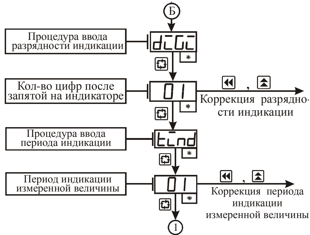
Рисунок 3.6 – Схема алгоритма работы в режиме “Коэффициенты” (продолжение)
