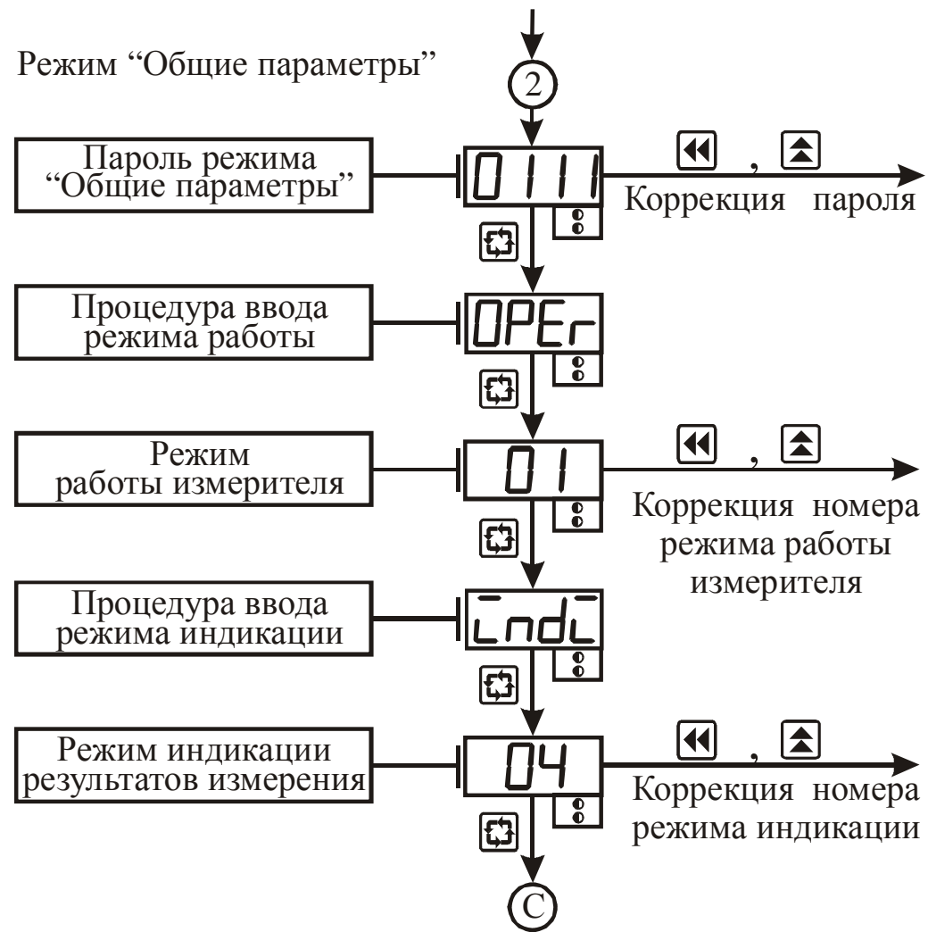
Рисунок 3.4 – Схема алгоритма работы прибора в режиме “Общие параметры”
