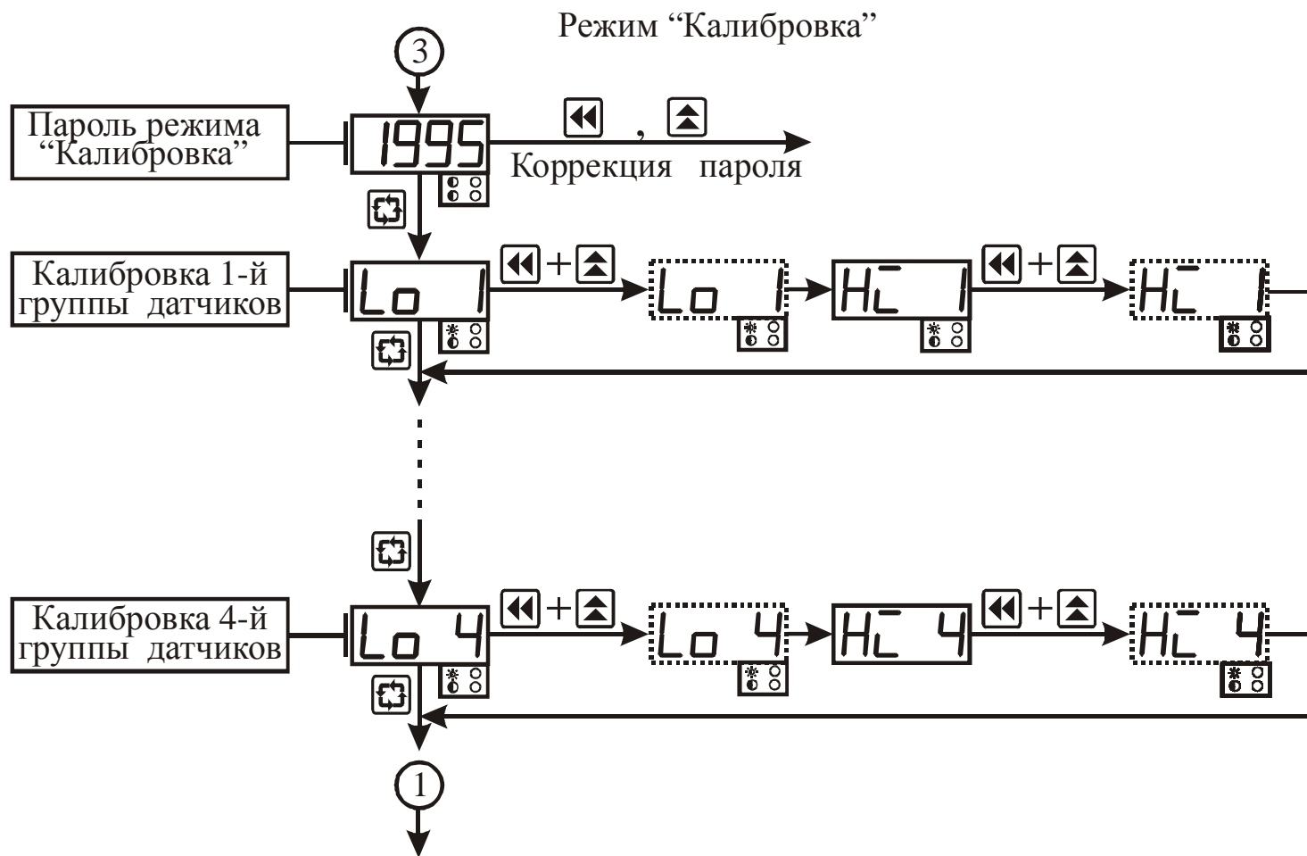
Рисунок 3.11 – Схема алгоритма работы в подрежиме “ Калибровка 1-го канала”
