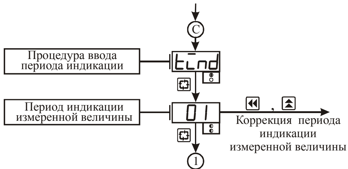
Рисунок 3.5 – Схема алгоритма работы прибора в режиме “Общие параметры (продолжение)”
