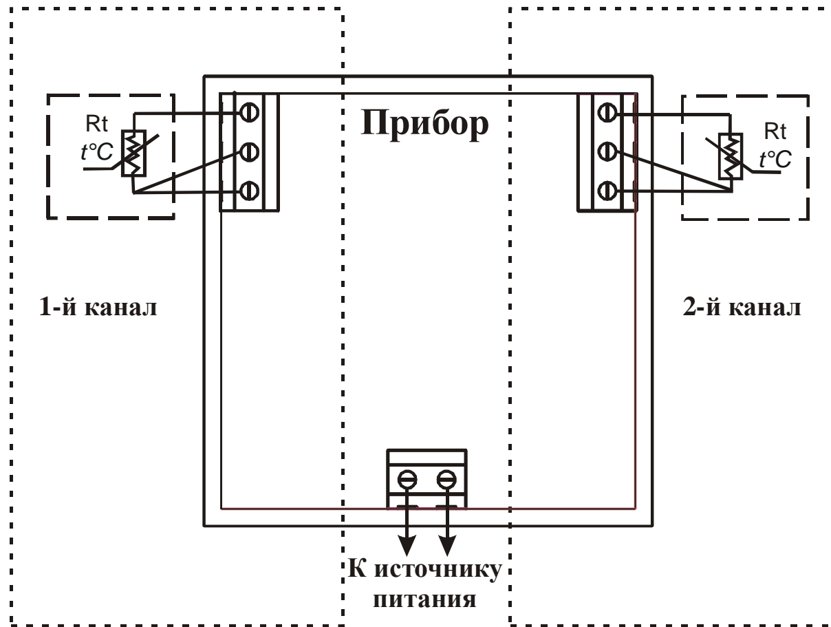
Рисунок 8.1 – Схемы подключения ТС и источника питания
