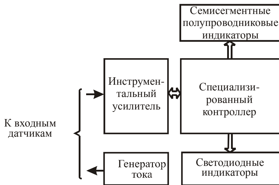
Рисунок 3.1 – Функциональная схема прибора
