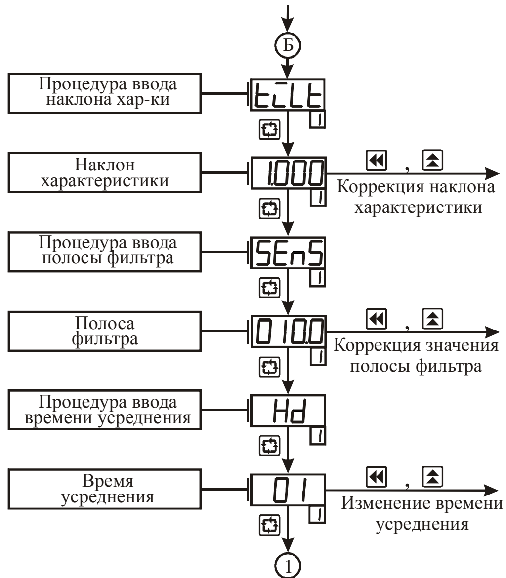
Рисунок 3.6 – Схема алгоритма работы в подрежиме “Коэффициенты 1-го канала” (окончание)
