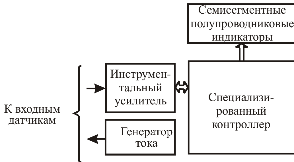
Рисунок 3.1 – Функциональная схема прибора
