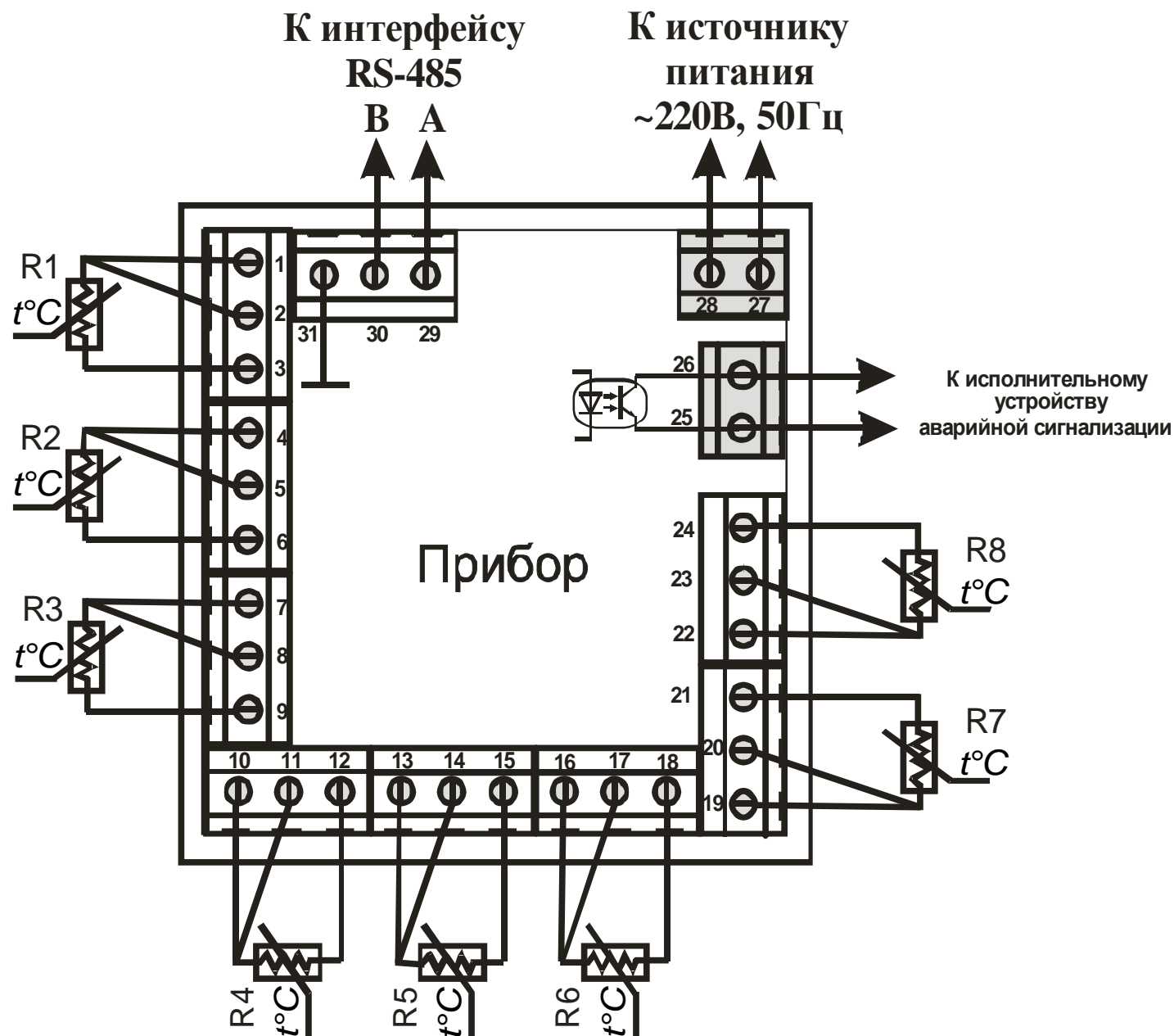
Рисунок 8.1 – Схема подключения ТС, интерфейса RS-485 и источника питания
