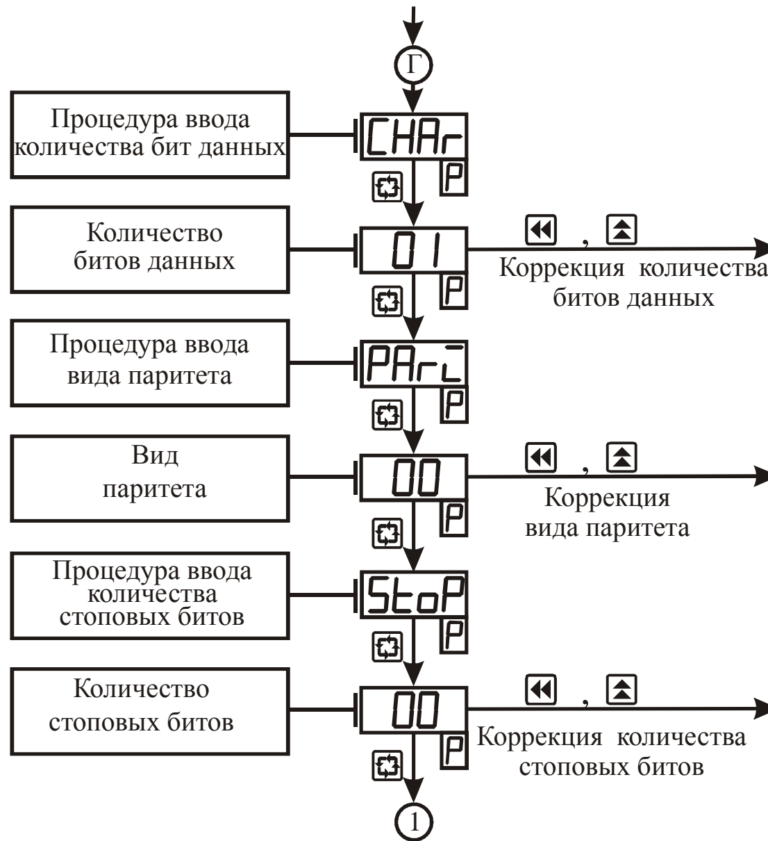
Рисунок 3.14 – Схема алгоритма работы в режиме “Настройка RS-485” (окончание)
