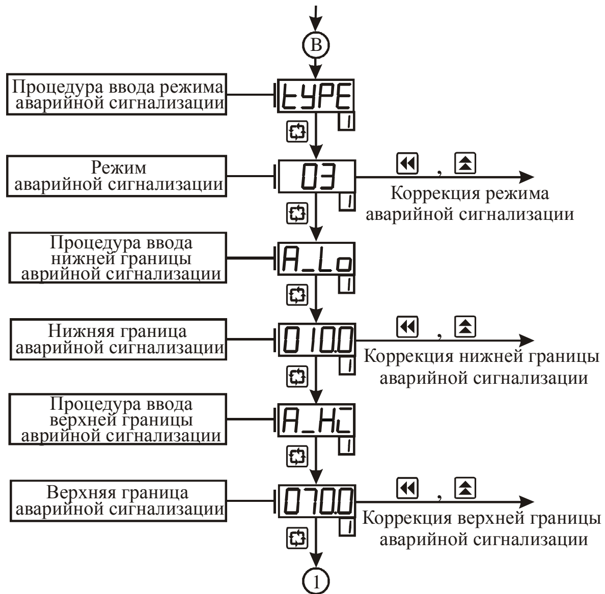
Рисунок 3.8 – Схема алгоритма работы в подрежиме “Коэффициенты 1-го канала” (окончание)
