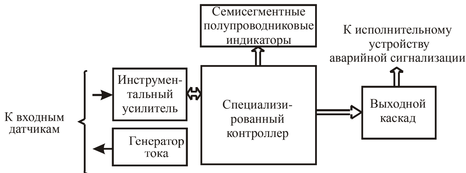
Рисунок 3.1 – Функциональная схема прибора
