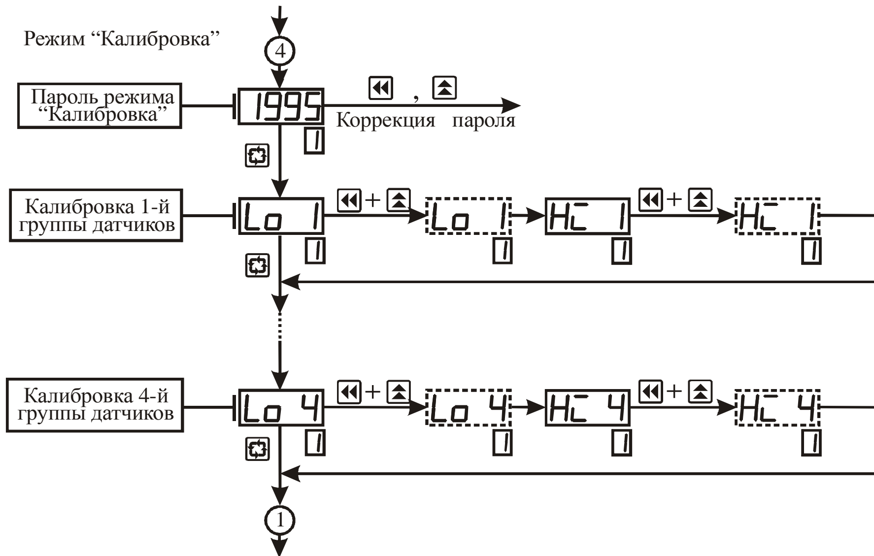
Рисунок 3.12 – Схема алгоритма работы в подрежиме “Калибровка 1-го канала”
