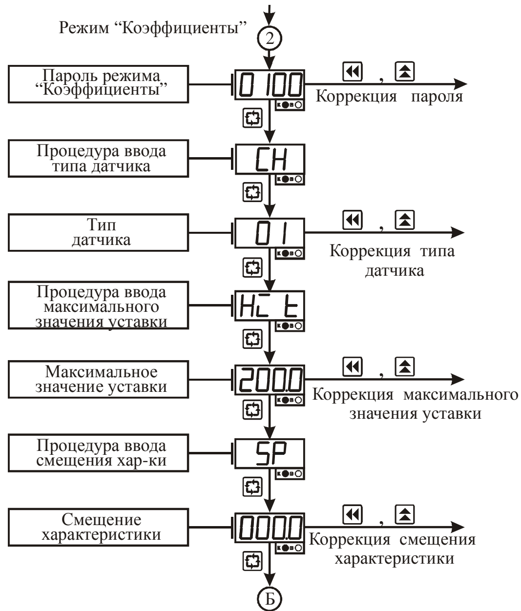
Рисунок 3.6 – Схема алгоритма работы в режиме “Коэффициенты”
