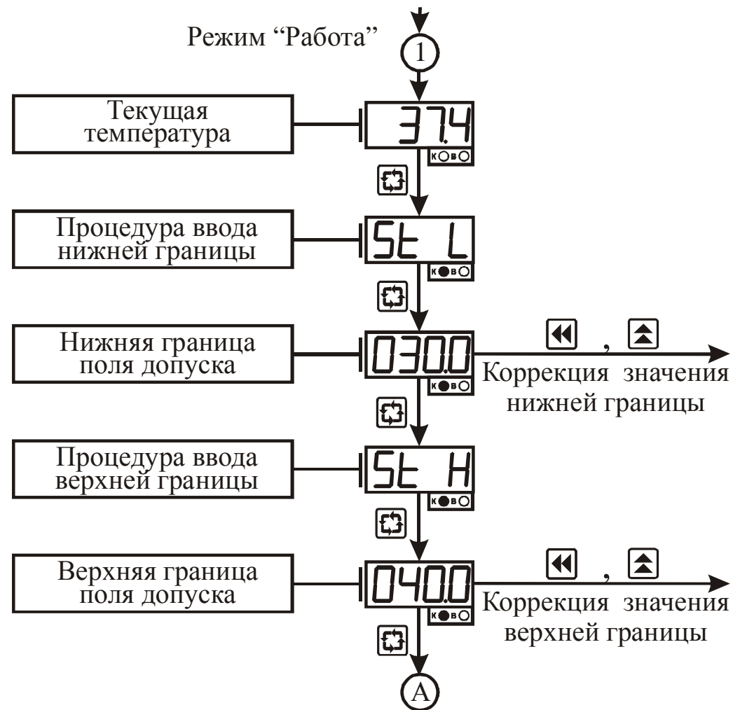
Рисунок 3.4 – Схема алгоритма работы прибора при типе логики работы выхода “03” и “04”
