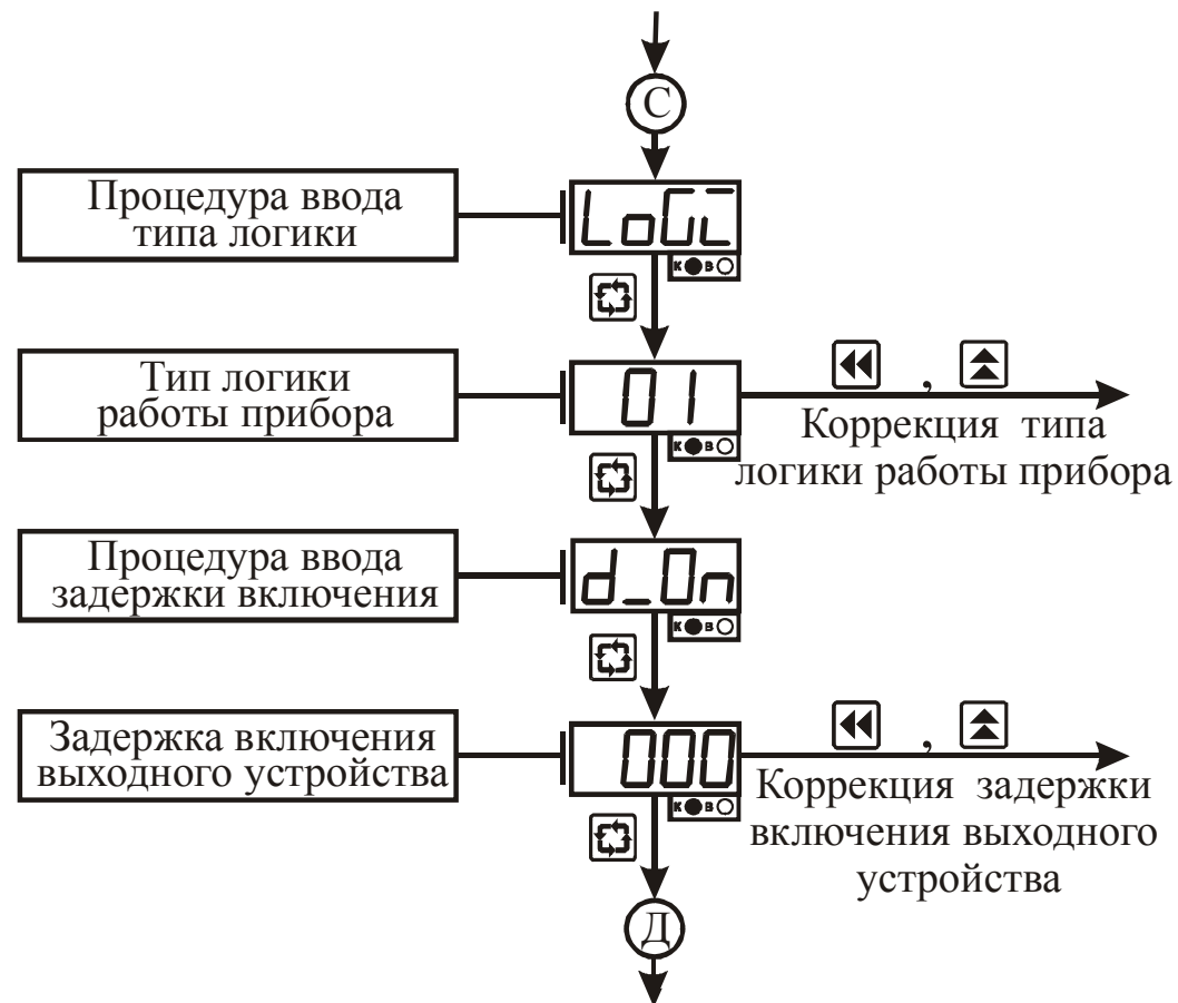
Рисунок 3.8 – Схема алгоритма работы в режиме “ Коэффициенты ” (продолжение)
