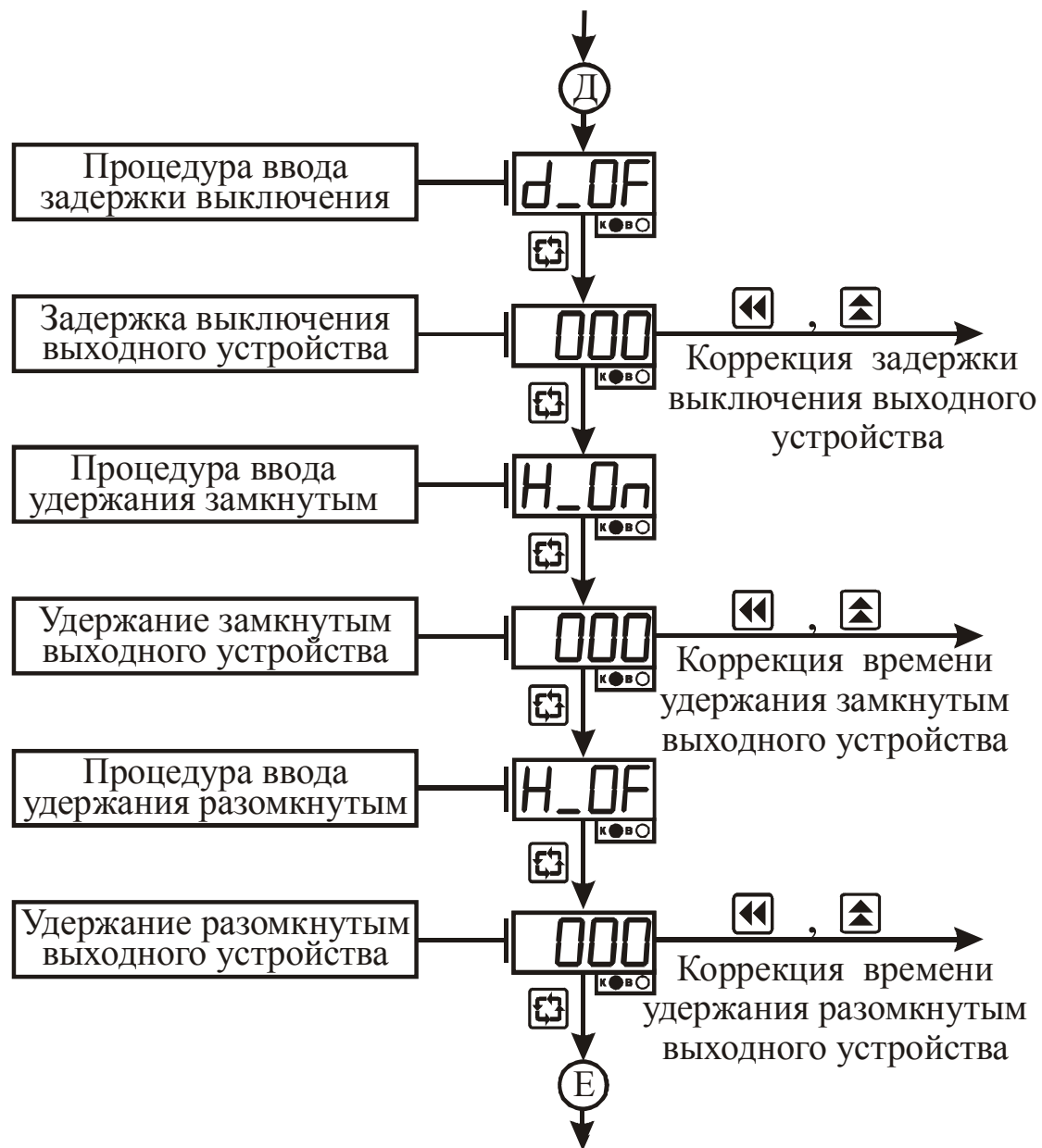
Рисунок 3.9 – Схема алгоритма работы в режиме “ Коэффициенты ” (продолжение)
