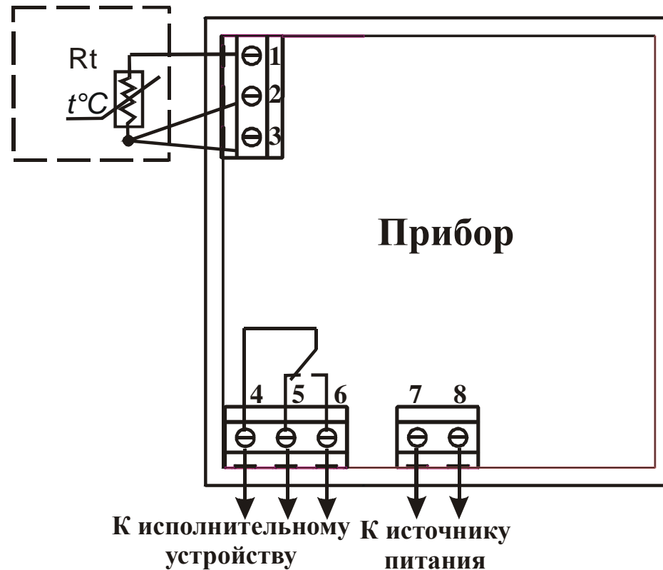
Рисунок 8.1 – Схемы подключения ТС, источника питания и исполнительного устройства
