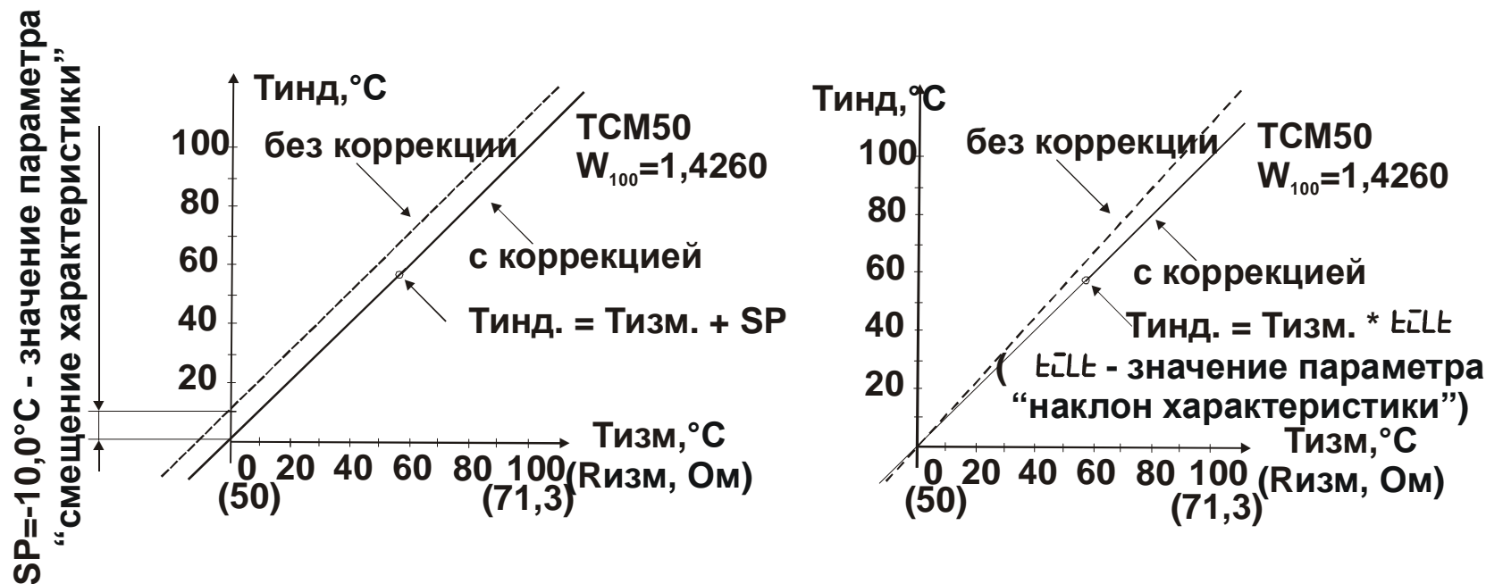
Рисунок 3.11 - Влияние параметров "Смещение характеристики" и "Наклон характеристики" на характеристику преобразования
