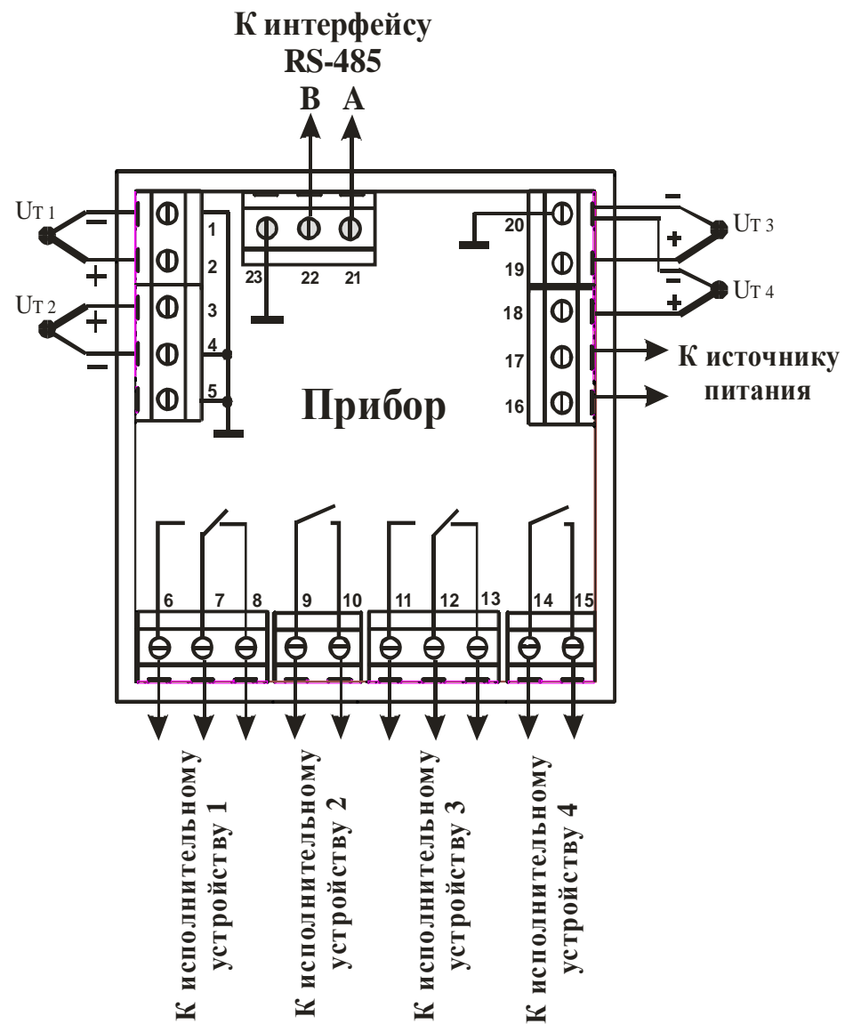
Рисунок 8.1 – Схема подключения ТТ, интерфейса RS-485, источника питания и исполнительных устройств
