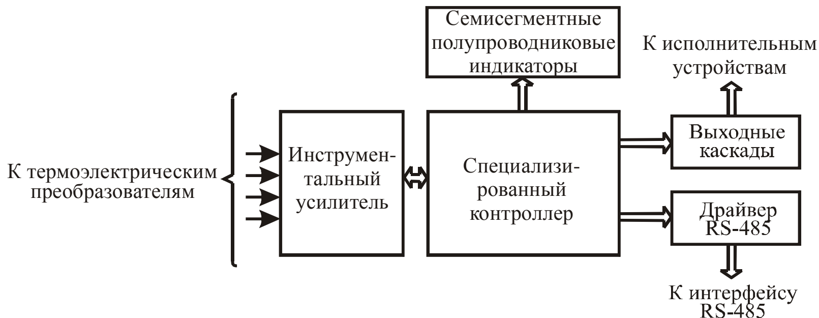
Рисунок 3.1 – Функциональная схема прибора
