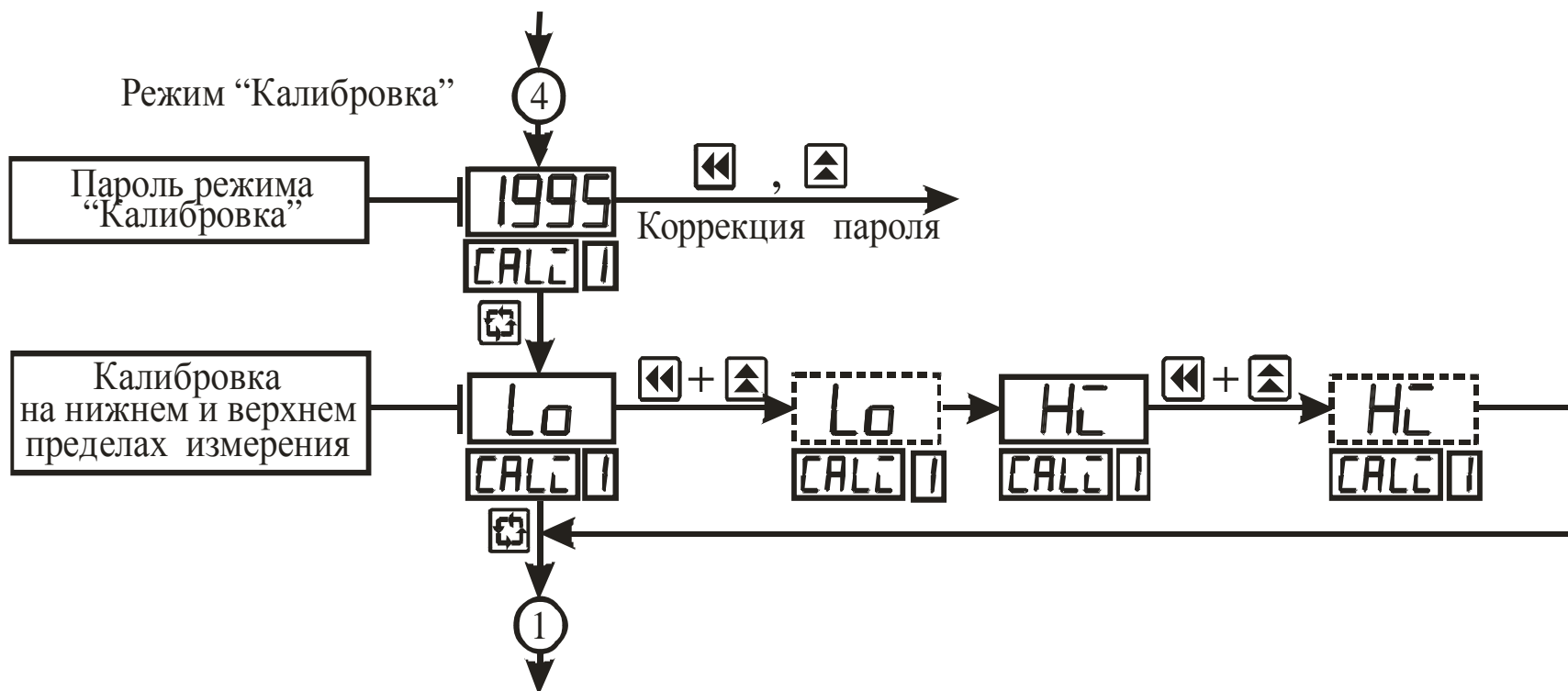
Рисунок 3.14 – Схема алгоритма работы в подрежиме "Калибровка 1-го канала"
