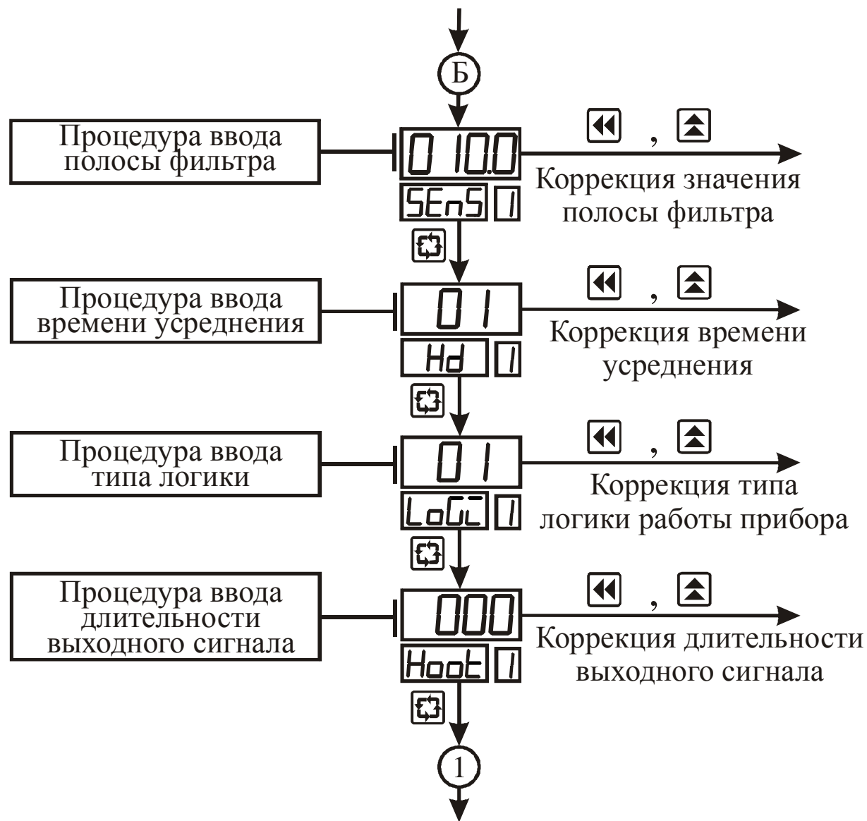
Рисунок 3.9 – Схема алгоритма работы в подрежиме “Коэффициенты 1-го канала” (окончание)
