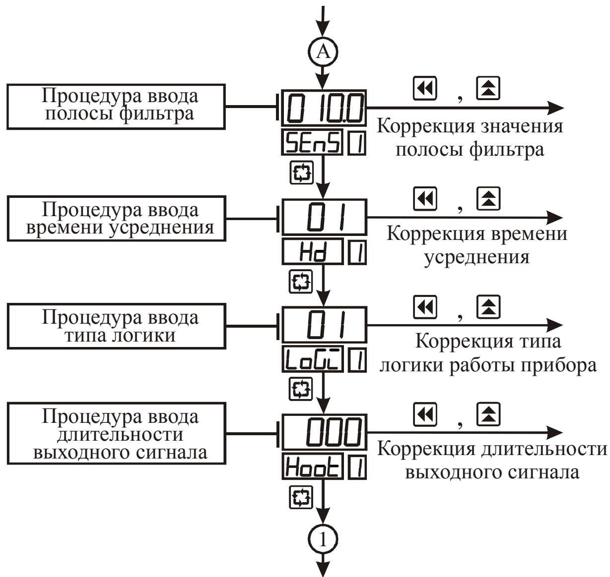
Рисунок 3.8 – Схема алгоритма работы в подрежиме “Коэффициенты 1-го канала” (окончание)
