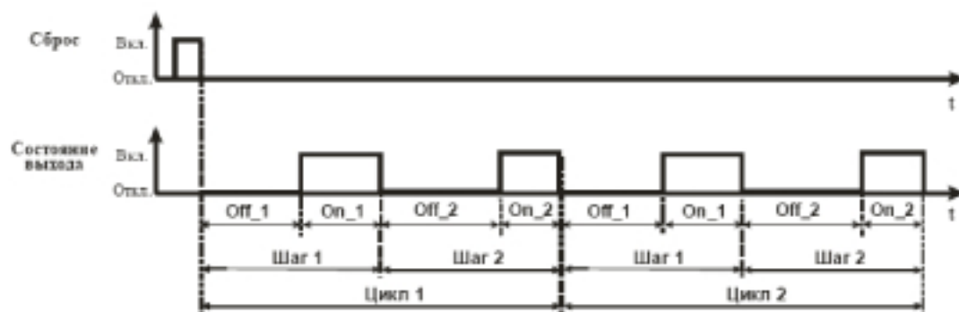
Рисунок 3.2 – Временная диаграмма работы прибора
