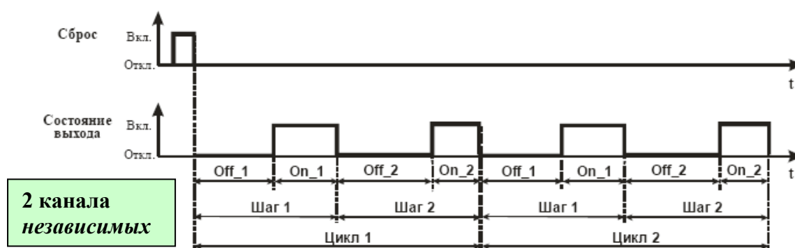
Рисунок 3.2 – Временные диаграммы работы прибора
