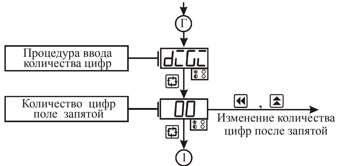
Рисунок 3.10 – Схема алгоритма работы в режиме “ Коэффициенты 1-го канала ” (окончание)
