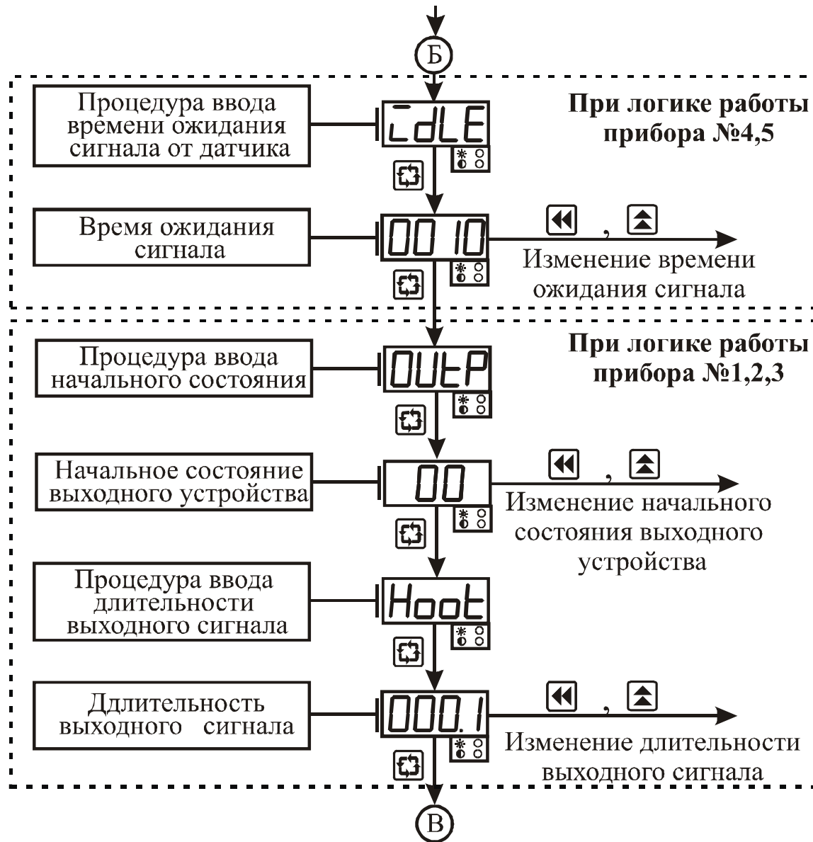
Рисунок 3.8 – Схема алгоритма работы в подрежиме “Коэффициенты 1-го канала” (продолжение)
