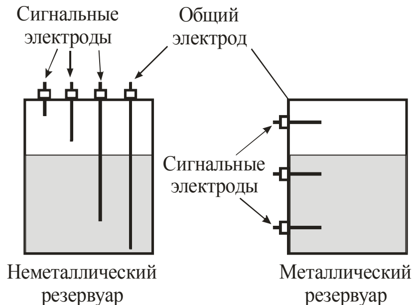
Рисунок 2.1 – Подключение датчиков уровня к объекту
