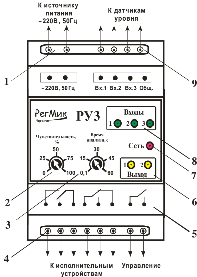
Рисунок 2.3 – Внешний вид прибора
