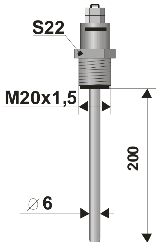
Рисунок 2.4 – Внешний вид и габаритные размеры датчика уровня
