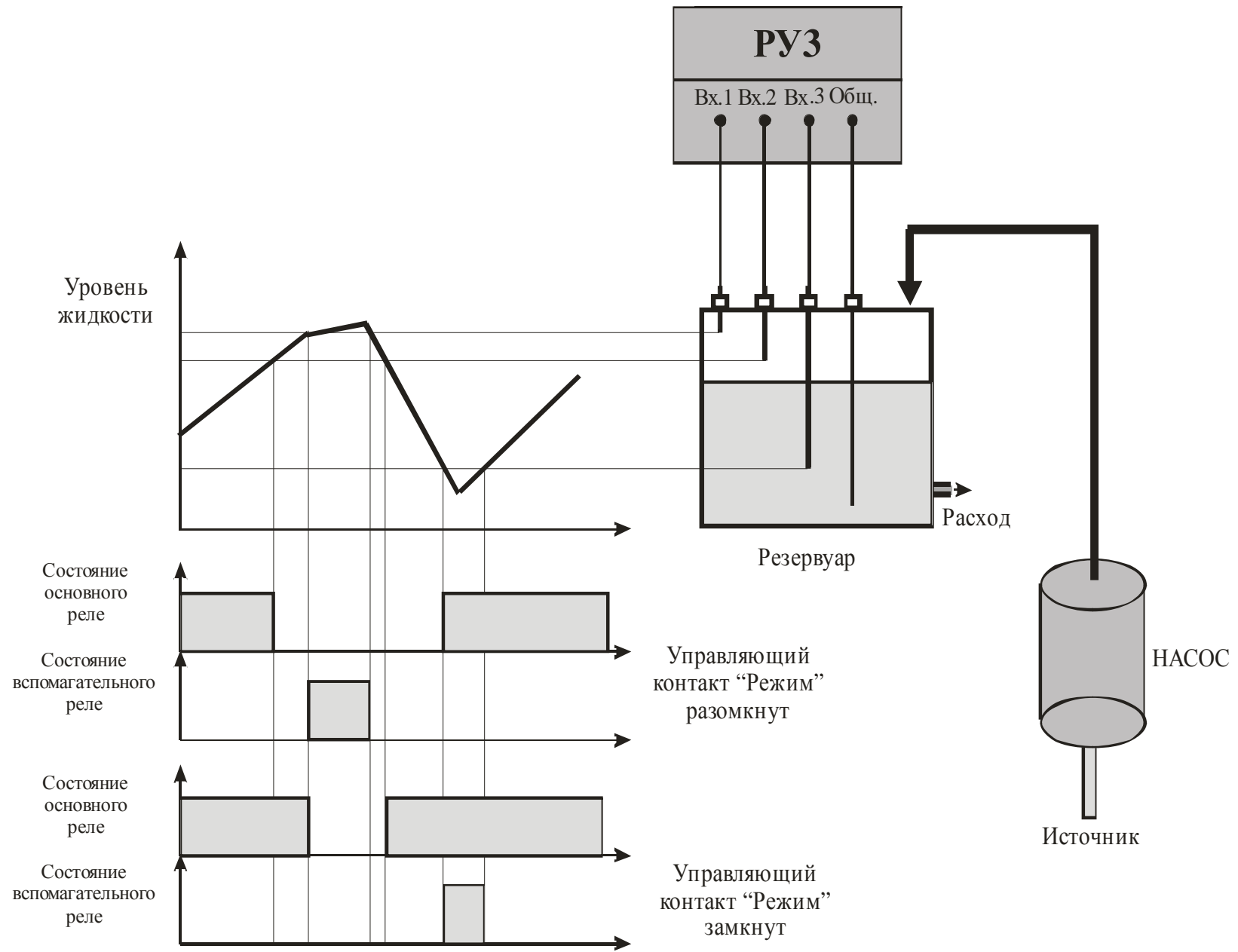
Рисунок 2.2 – Временные диаграммы работы прибора
