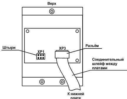
Рис. 5. Расположение коммутатора XP1. Вид обратной стороны передней платы монитора при снятой крышке
