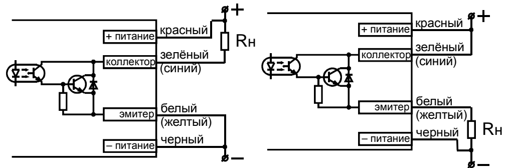
Рис.2. Схемы подключения фотодатчика МикРА Ф2.
